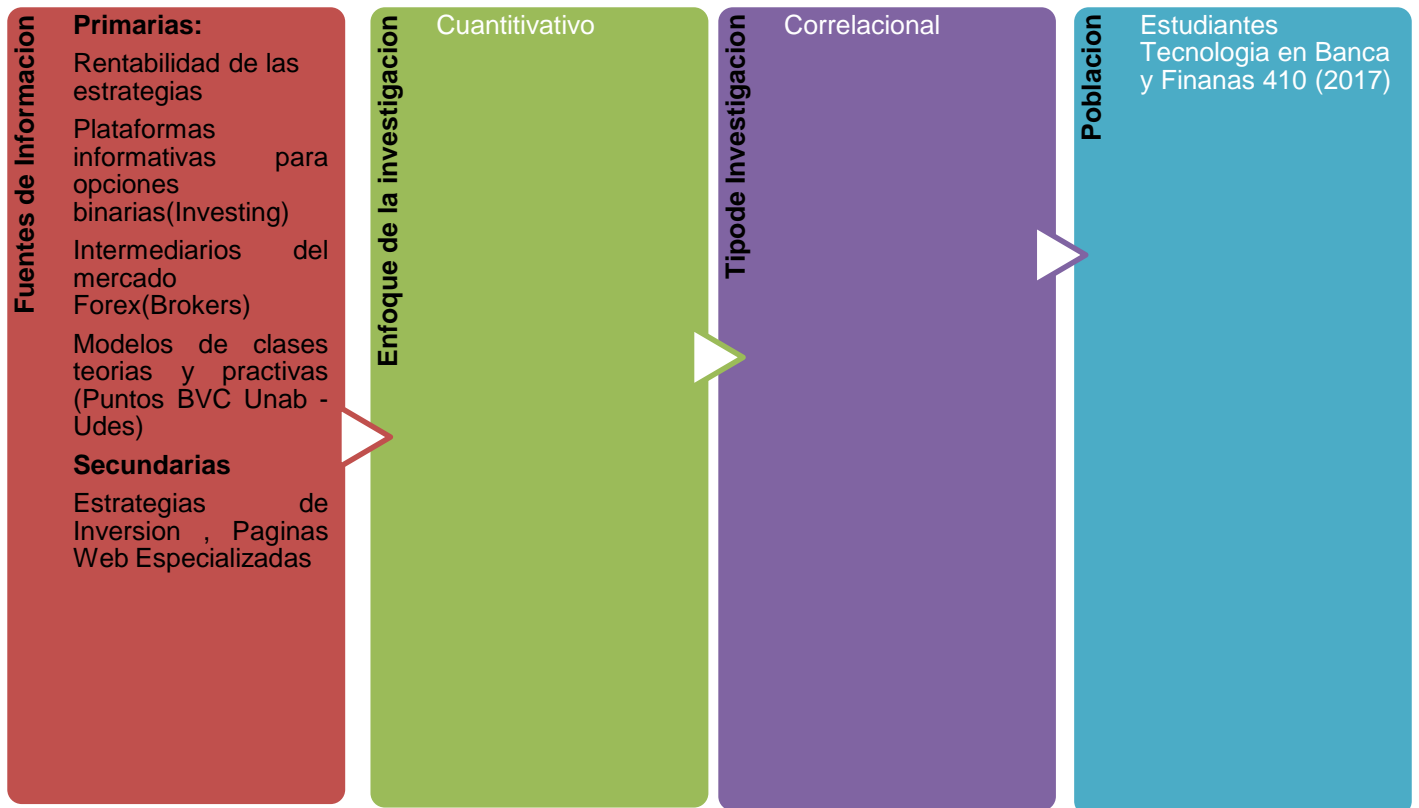
Ilustración 2: Metodología Propuesta
