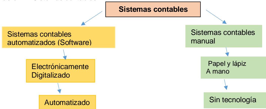
Ilustración 1: Sistemas contables
