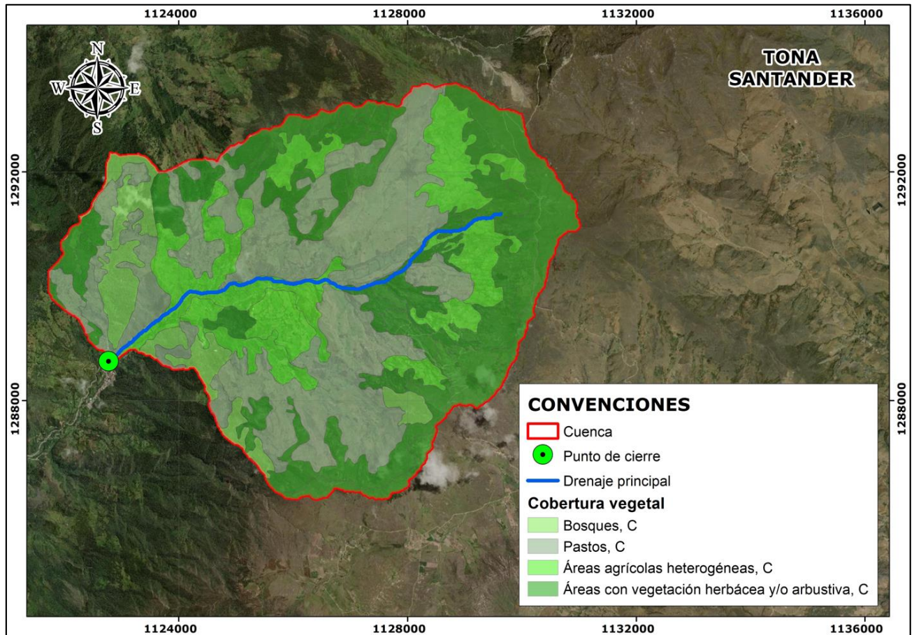
Imagen 5. Número de curva cuenca hidrográfica.
