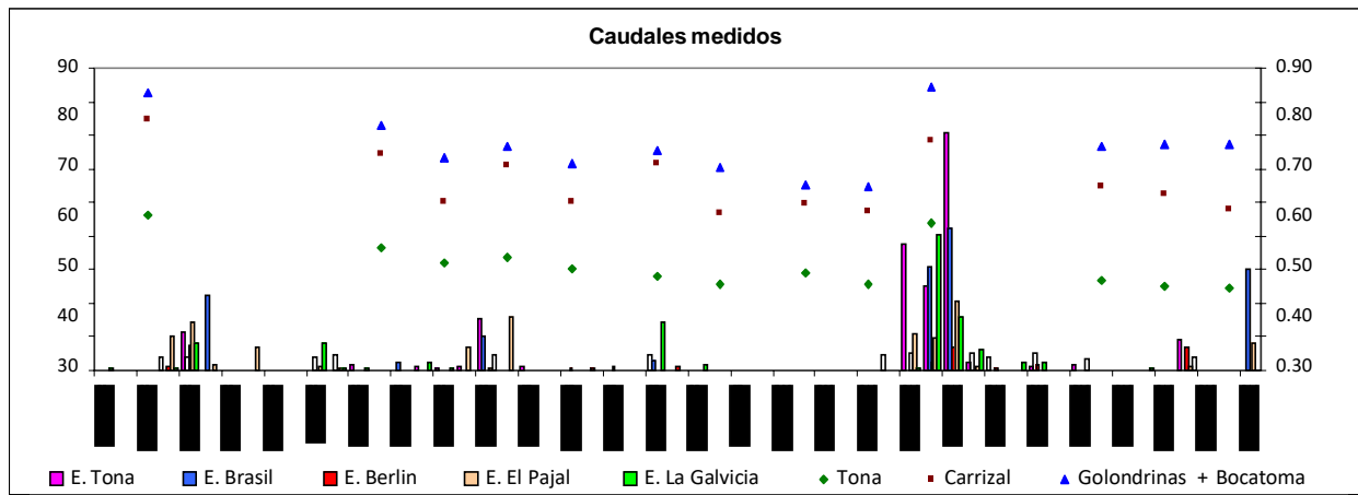
Ilustración 18. Caudales medidos en las estaciones sobre el río Tona
