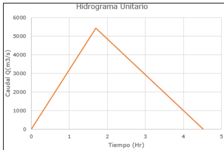
Imagen 6. Hidrograma unitario triangular.
