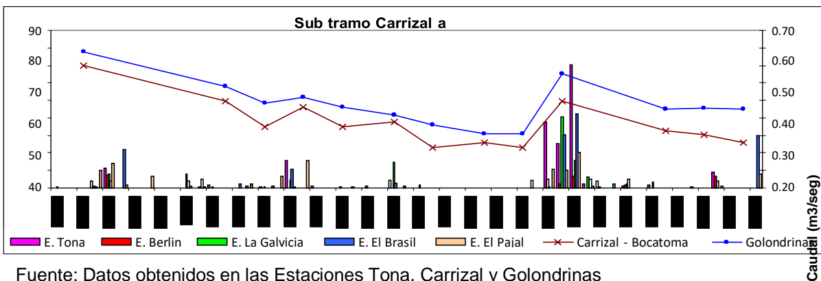
Ilustración 23. Caudal de Carrizal – caudal captado Bocatoma vs caudal Golondrinas
