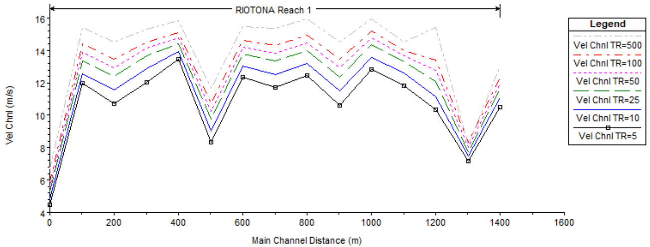
Imagen 11. Distribuciones de velocidades.
