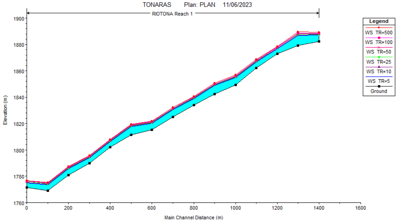
Imagen 10. Perfil longitudinal del modelo.
