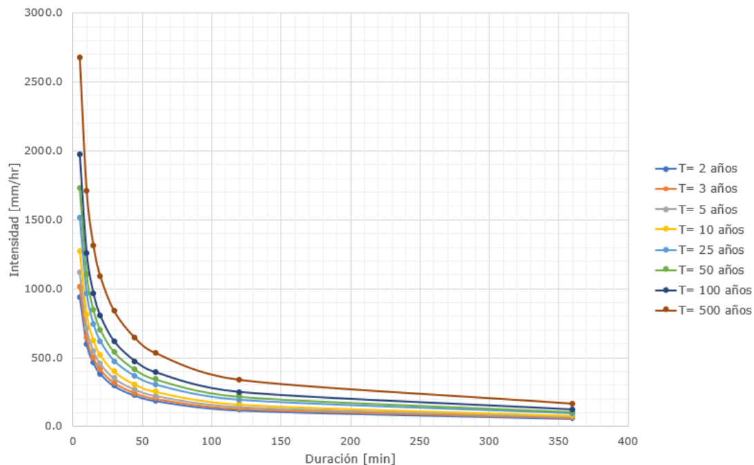
Imagen 4. Curva IDF intensidad (mm/hr) vs duración (min).
