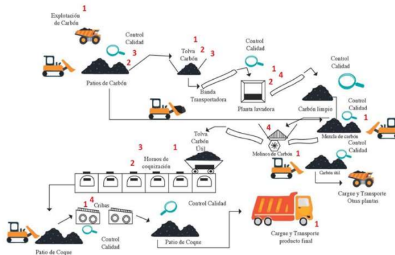
Figura 2. Etapas obtención del Coque
