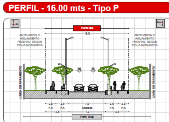
Figura 35, Perfil 16.00 Tipo P
