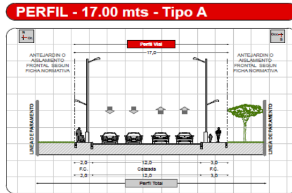
Figura 36, Perfil 17.00 Tipo A
