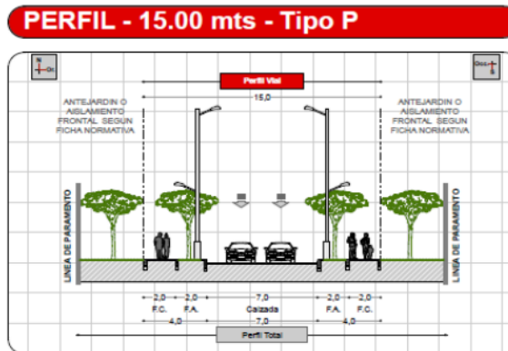
Figura 34, Perfil 15.00 Tipo P
