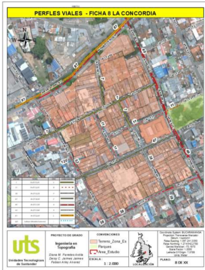
Figura 31, Perfiles Viales POT
