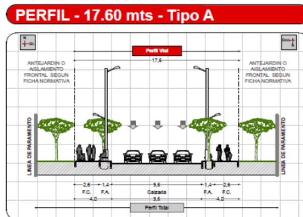
Figura 37, Perfil 17.60 Tipo A
