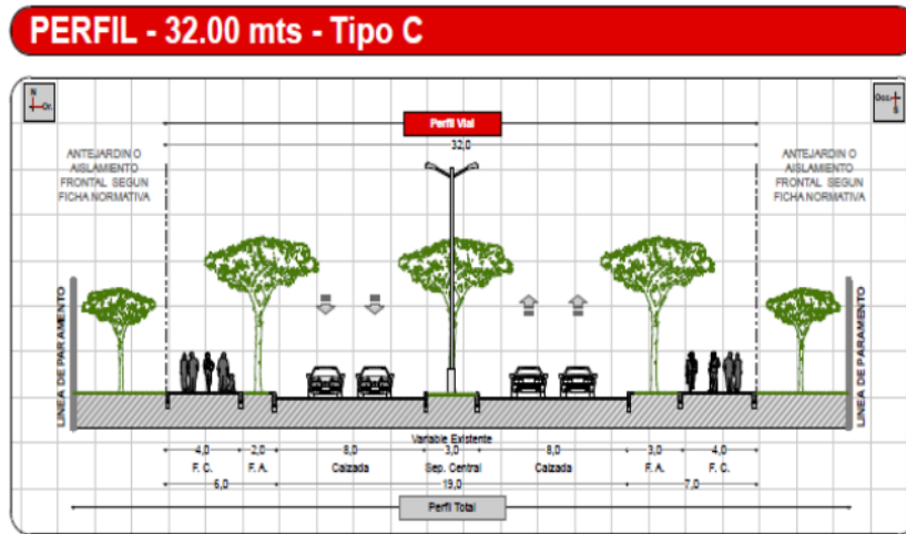
Figura 38, Perfil 32.00 Tipo C
