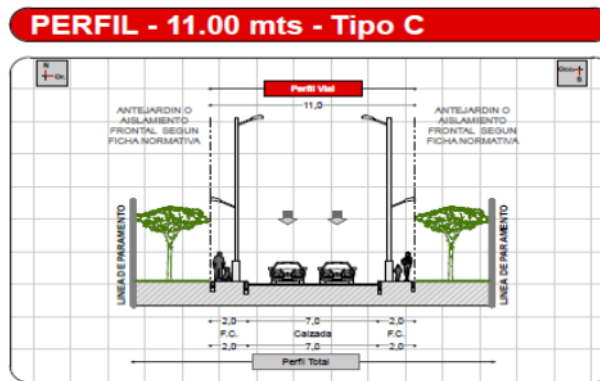
Figura 32, Perfil 11.00 Tipo C
