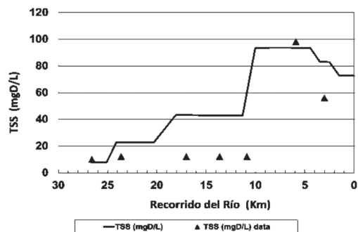
Figura 8. Modelado de los sólidos totales en el río Frío.
