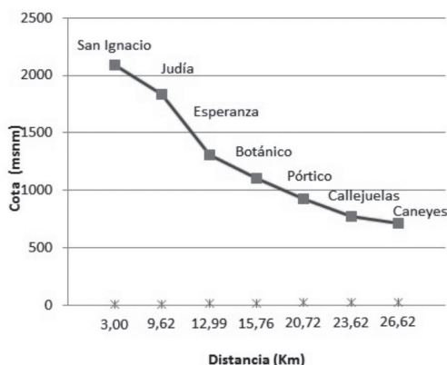
Figura 2. Perfil longitudinal de altura- R Frío.
