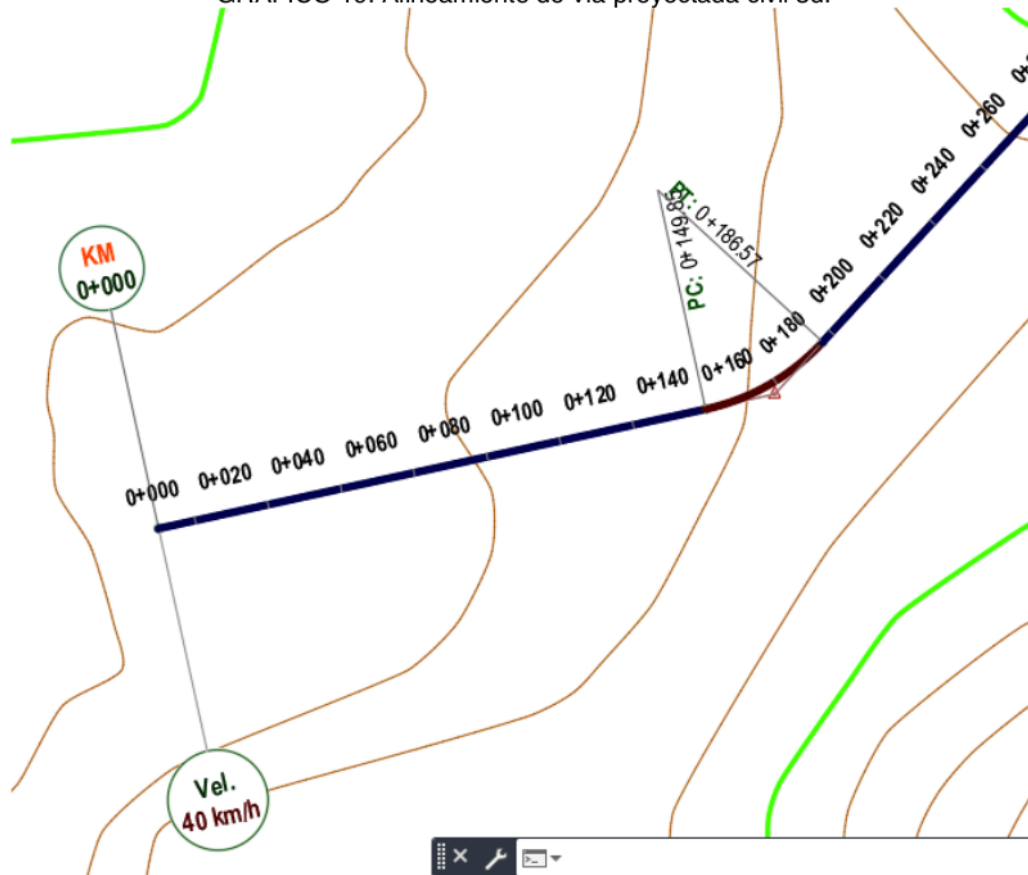
GRAFICO 19. Alineamiento de vía proyectada civil 3d.
