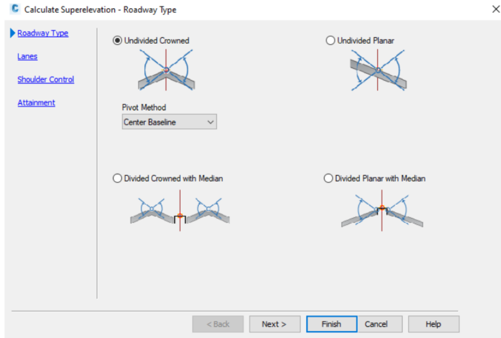
GRAFICO 31. Parámetros de vía
