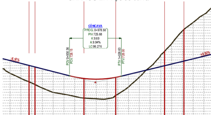
GRAFICO 27. Tipo de curva
