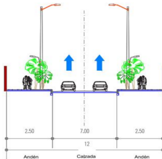
GRAFICO 7. Perfil vial
