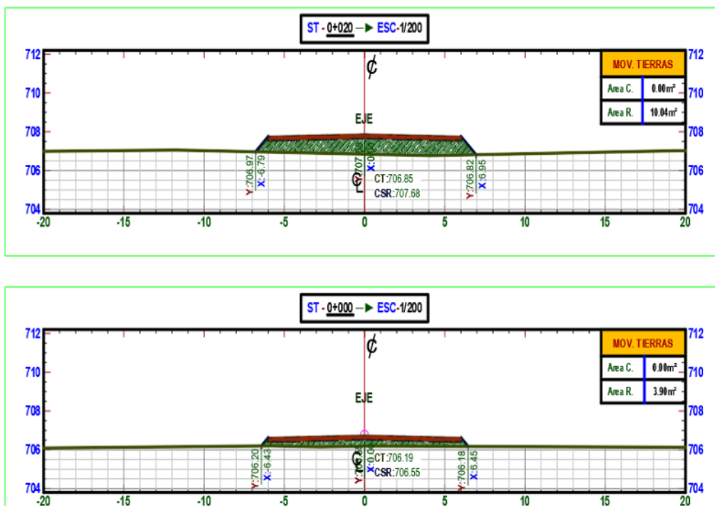
GRAFICO 41. Secciones transversales
