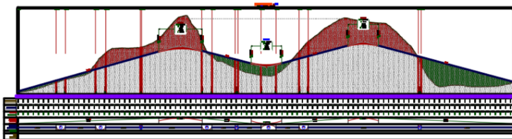
GRAFICO 29. Perfil con cortes y rellenos
