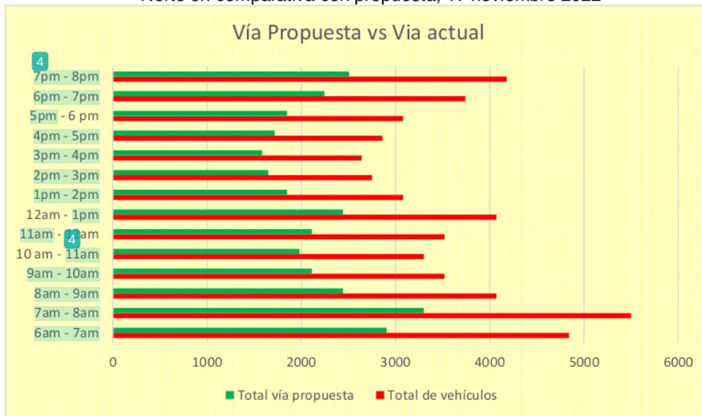
GRAFICO 50. Variación horaria del volumen de tránsito, vía rincón de girón, sentido sur – Norte en comparativa con propuesta, 17 noviembre 2022
