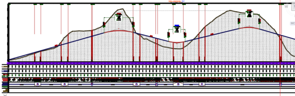
GRAFICO 26. Perfil de rasante
