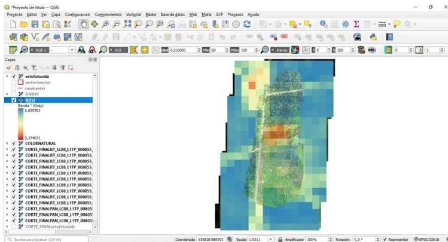
Figura 50. NDVI.
