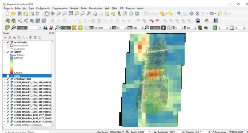
Figura 52. GNDVI.
