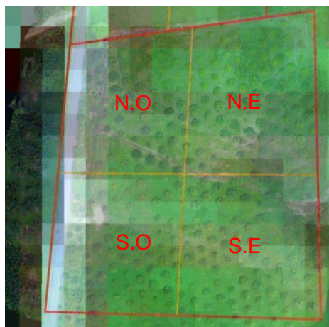
Figura 60. Sector 3.
