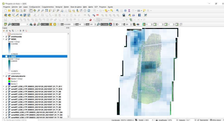
Figura 56. NDWI.
