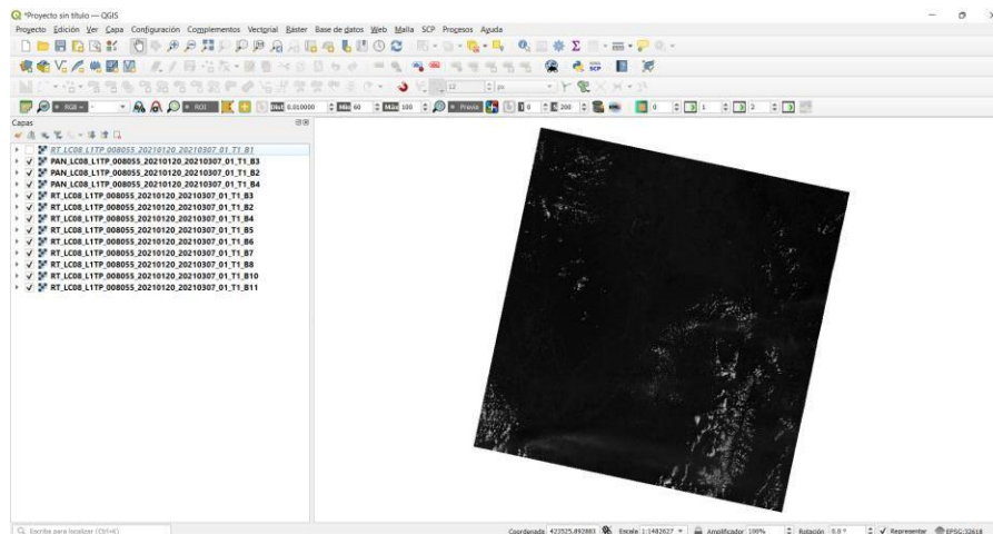
Figura 40. Bandas corregidas.
