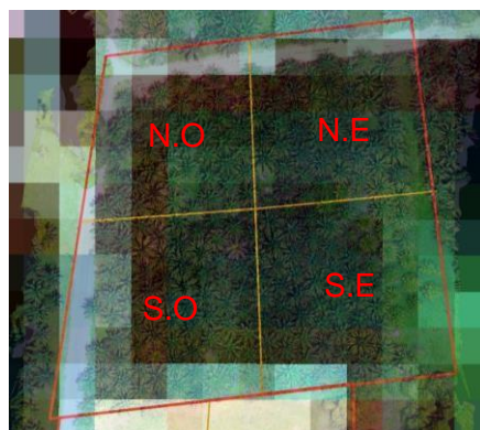
Figura 58. Sector 1.
