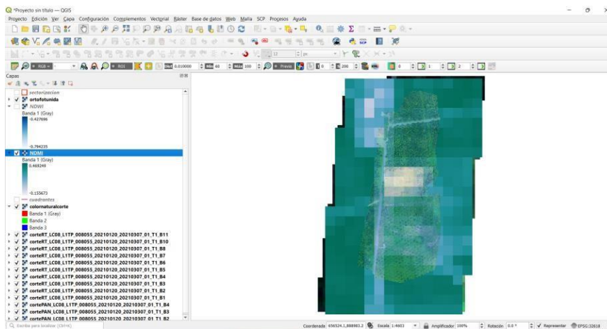
Figura 54. NDMI.
