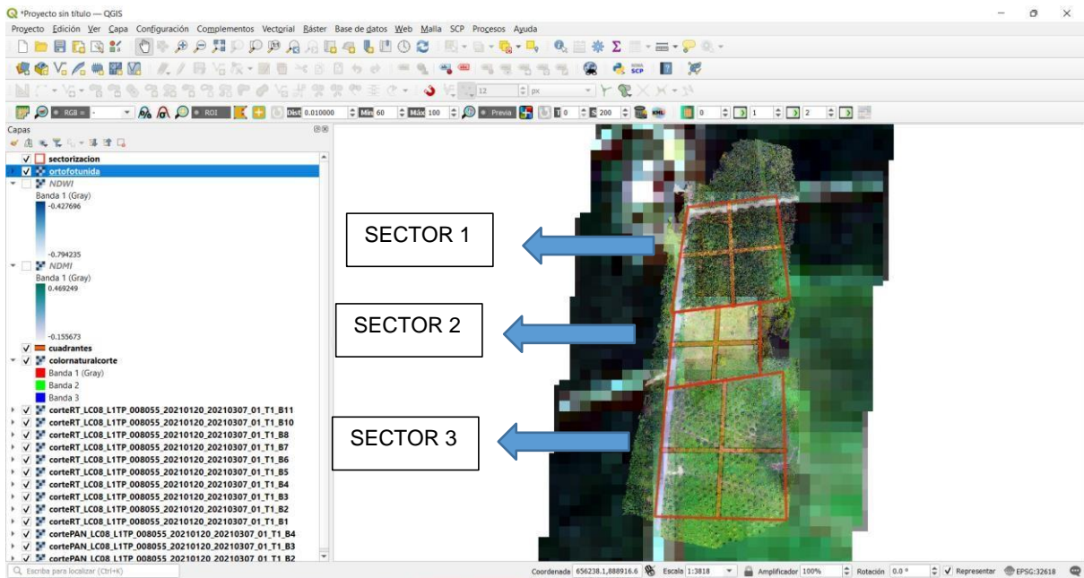
Figura 57. Sectorización.
