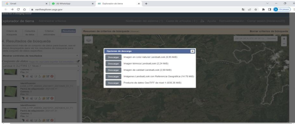
Figura 21. Imagen Landsat.
