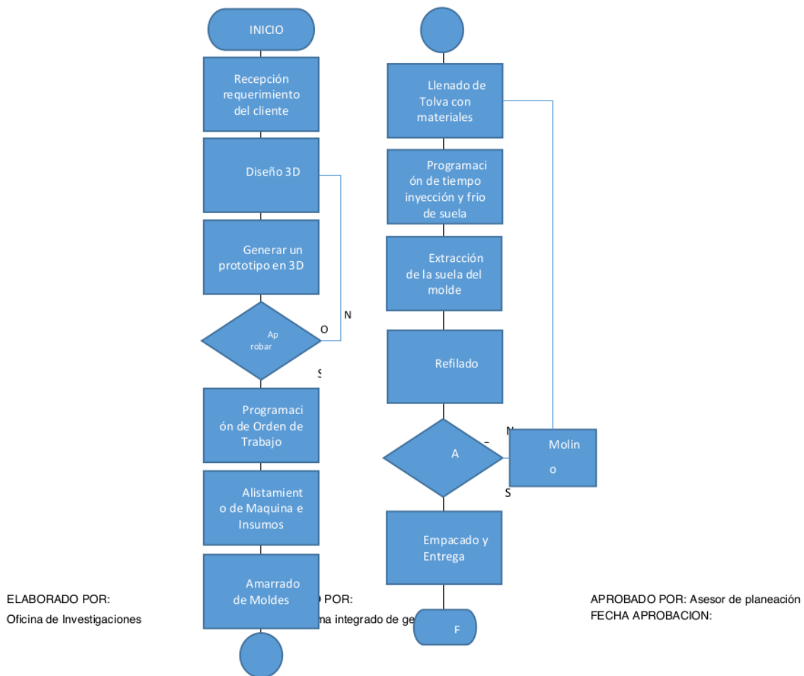
Figura 2. Diseño y elaboración de la suela PVC personalizada
