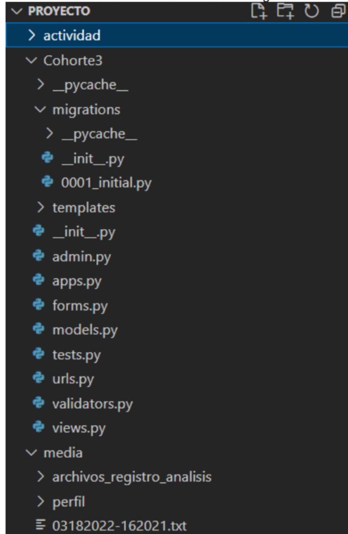
Ilustración 2 Estructura de código
