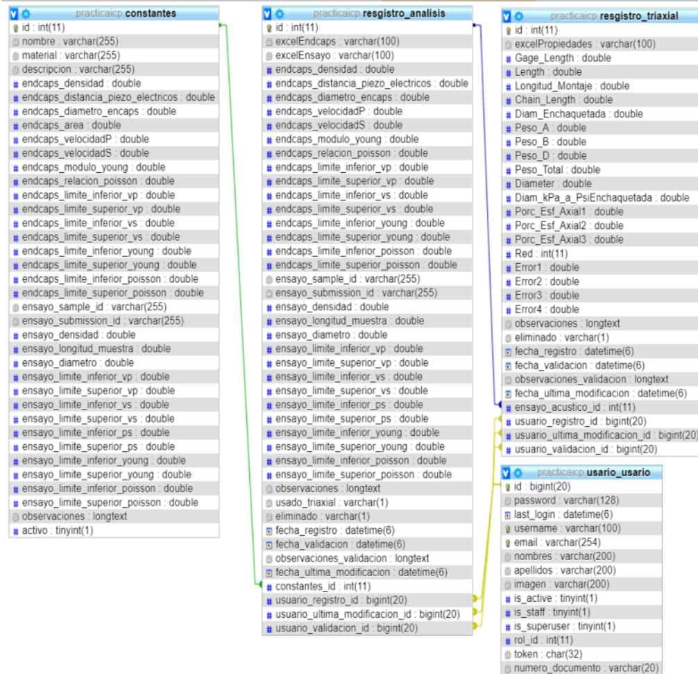
Ilustración 1 Modificación de la base de datos
