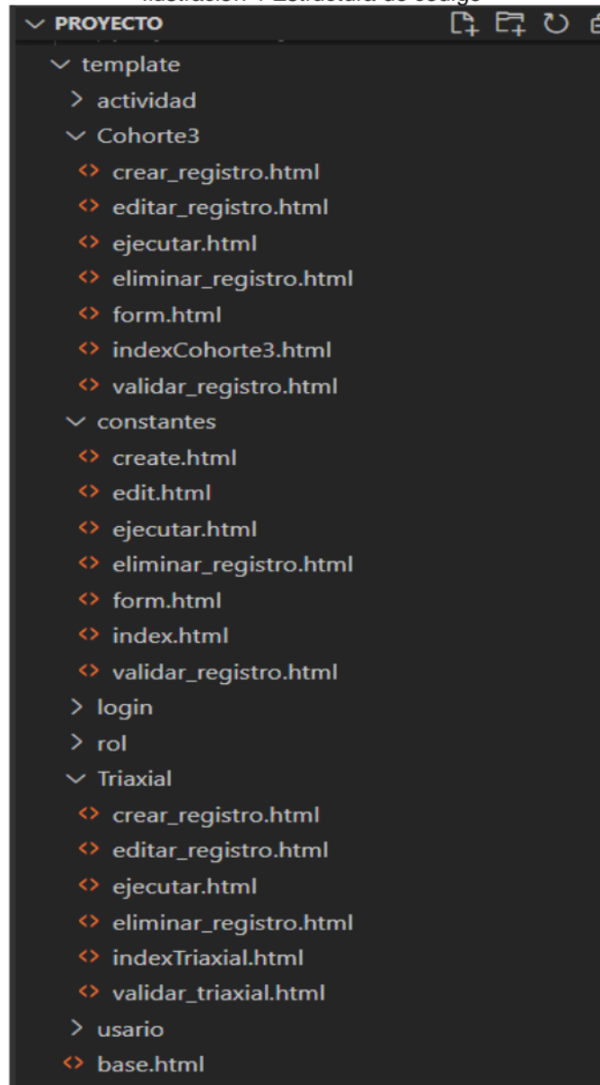
Ilustración 4 Estructura de código
